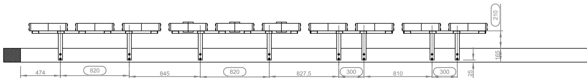
SCHNITT B-B
